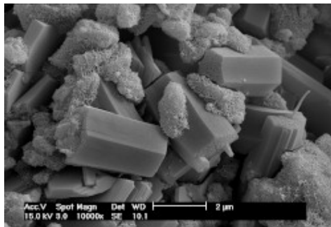
Hydratace Ultracoloru Plus, který obsahuje speciální pojivo na bázi hydraulických pojiv. Všimněte si tyčinkových krystalů hydroxidu vápenatého, který způsobuje výkvěty
